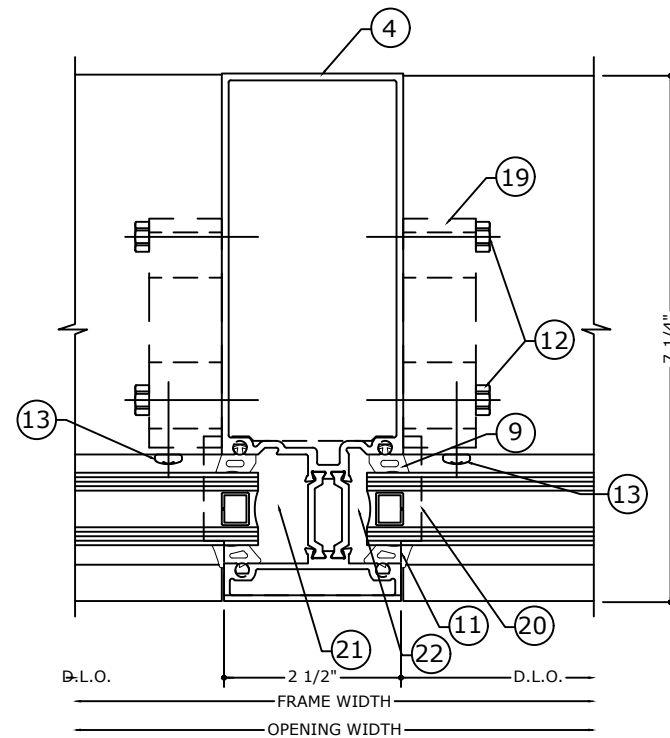
5 VERTICAL DETAIL - M1 SCALE: 6" = 1'-0"
