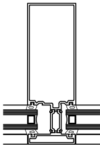
M1 DETAIL 4.1
