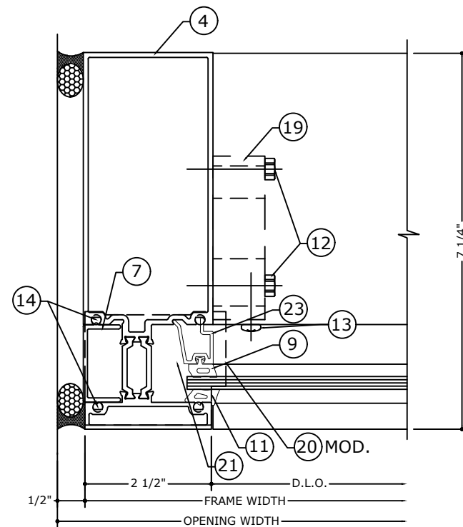
4.1 JAMB DETAIL - J1 SCALE: 6" = 1'-0"
